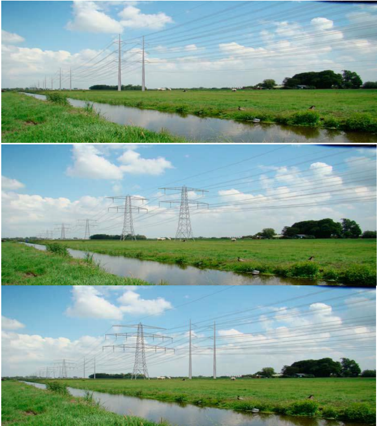
Figuur B2. Afbeeldingen (van boven naar beneden): Een gecombineerde vier-circuits bipole-mast; een twee-circuits vakwerkmast gebundeld met twee-circuits vakwerkmast; en een vier-circuits vakwerkmast gebundeld met twee-circuits bipole-mast. Bron: Startnotitie milieueffectrapportage Noord-West 380 kV.
