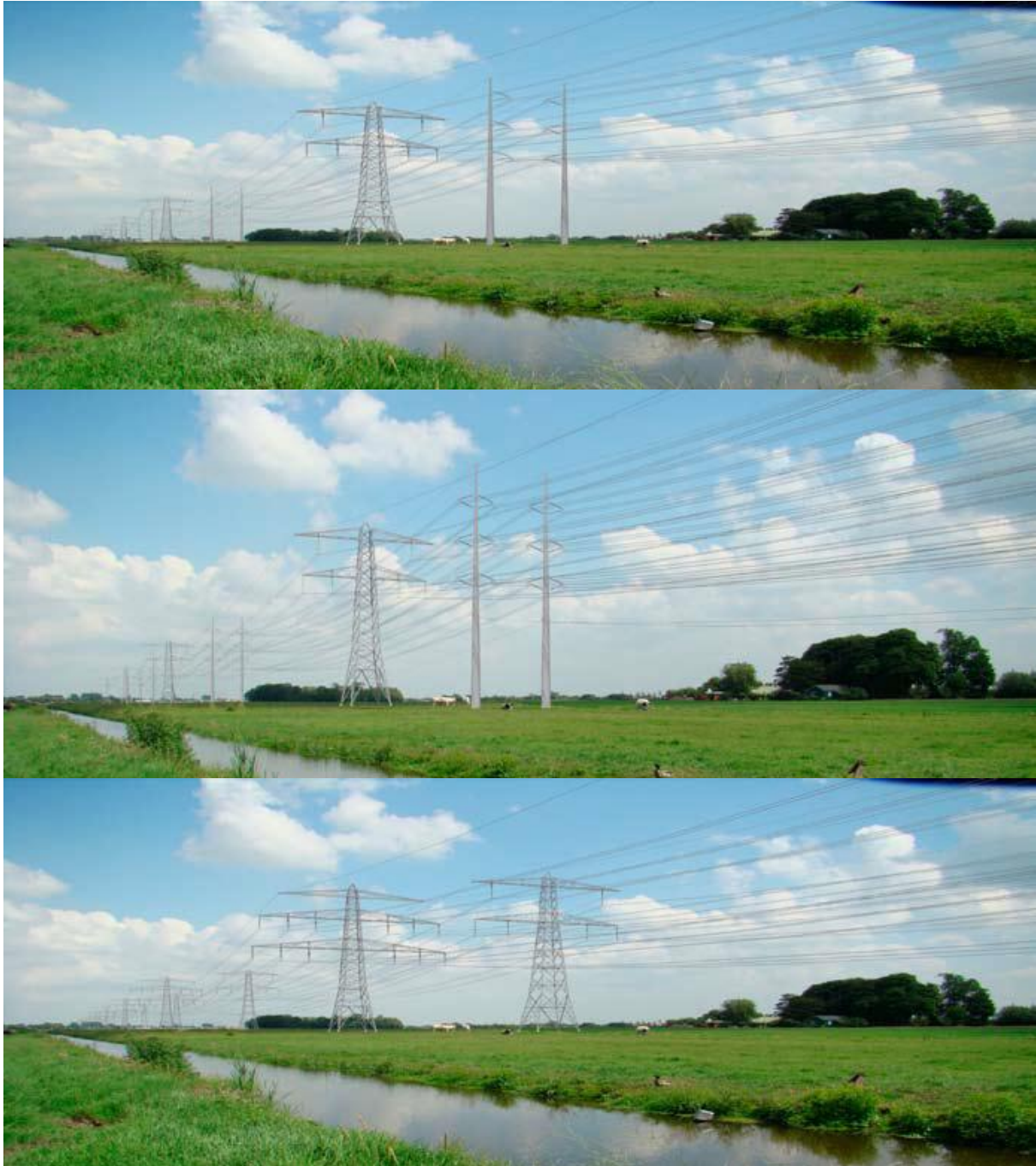
Figuur B3: Afbeeldingen van boven naar beneden: een twee-circuits vakwerkmast gebundeld met twee-circuits bipole-mast; een twee-circuits vakwerkmast gebundeld met een vier-circuits bipolemast; en een vier-circuits vakwerkmast gebundeld met twee-circuits vakwerkmast. Bron: Startnotitie milieueffectrapportage Noord-West 380 kV.
