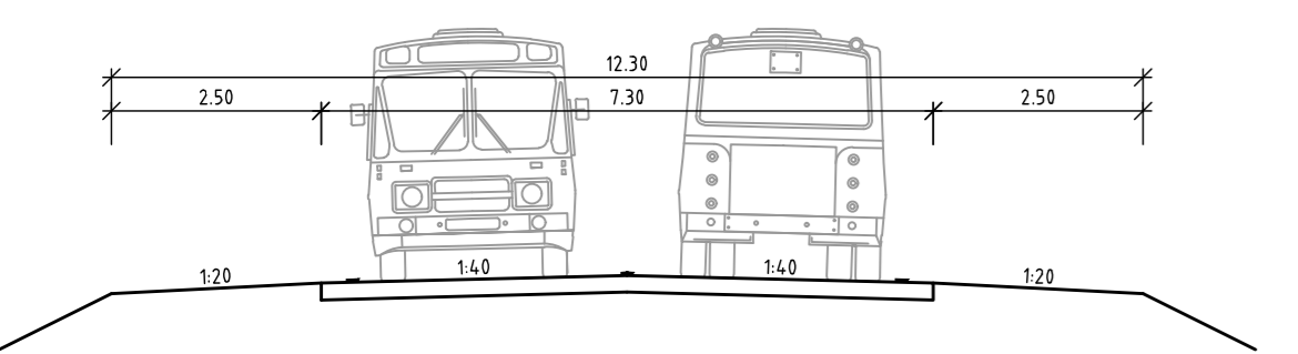
PRINCIPEPROFIEL 1A SCHAAAL 1:100 PROFIEL DOOR WONGEBIED TEN NOORDEN VAN LISSERWEG - IJWEG
