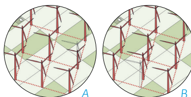
Grid A: Incidentele afwijking in de hoogte B: Incidentele afwijking in het stramien
