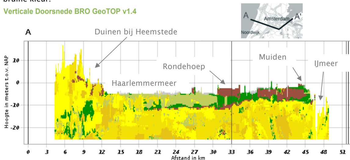
Figuur 8 dwarsdoorsnede
